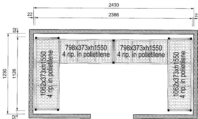
Boven aanzicht
